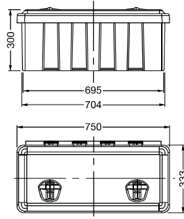
Trailer Tool Box 42 Liters Dorse Alet Çantası 42 Litre
